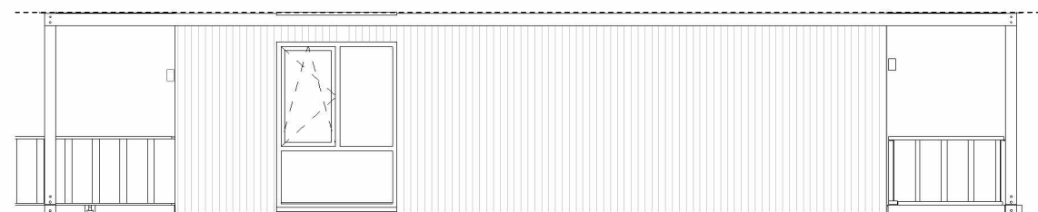
zijgevel
